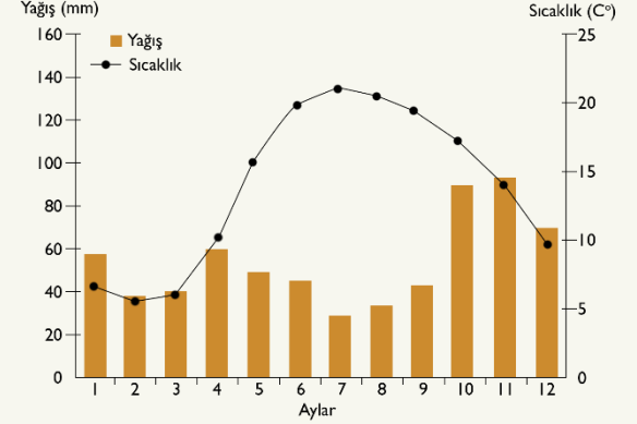
Samsun ili sıcaklık ve yağış grafiği
