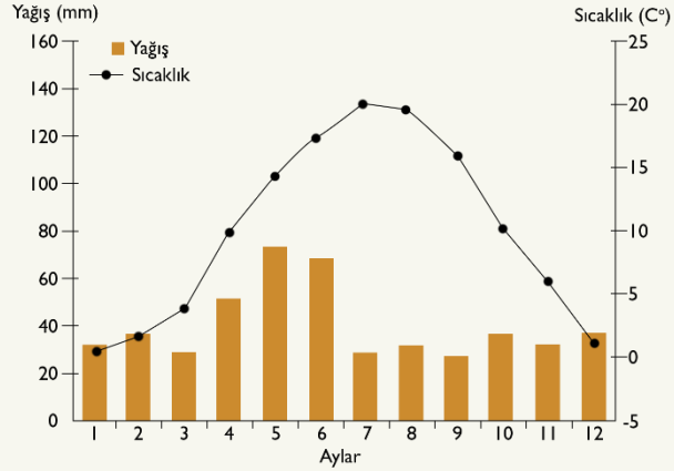
Kastamonu ili sıcaklık ve yağış grafiği
