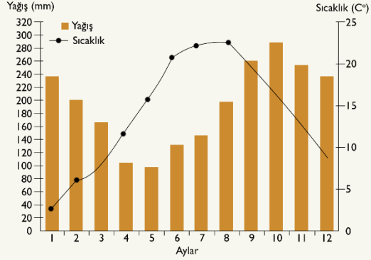
Rize ili sıcaklık ve yağış grafiği
