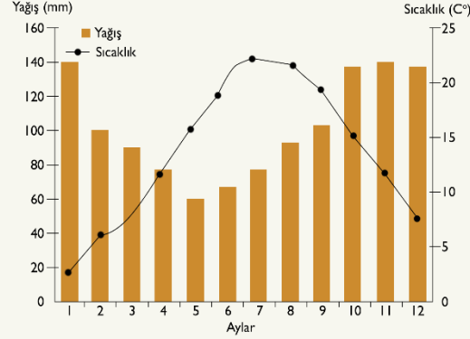
Zonguldak ili sıcaklık ve yağış grafiği
