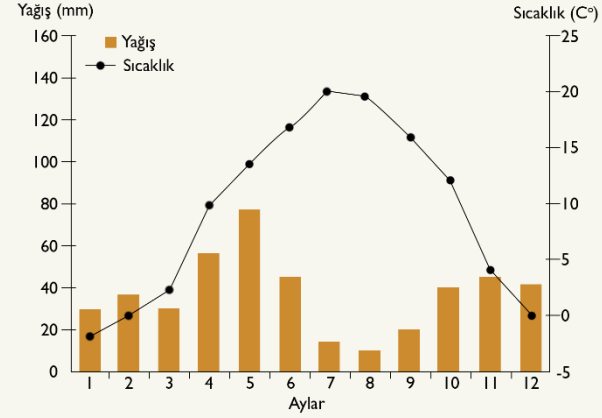
Gümüşhane ili sıcaklık ve yağış grafiği
